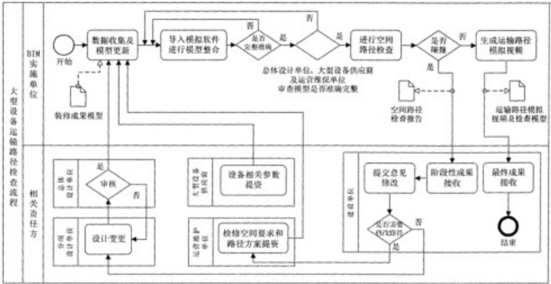
图 7 大型设备运输路径检查流程图
