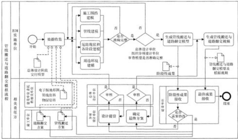
图 2 管线搬迁与道路翻交模拟流程图
